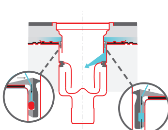
Mekaanisesti kiinnitetty laippa
