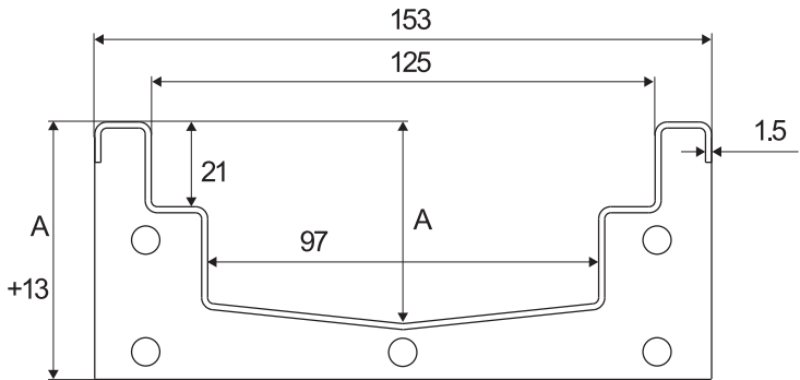
ACO lattiakouru 125 poikkileikkaus
