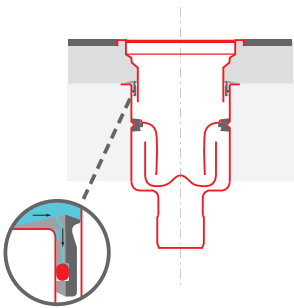
Paikannuslaippa
