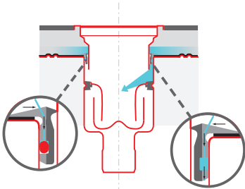
Liimattu laippa
