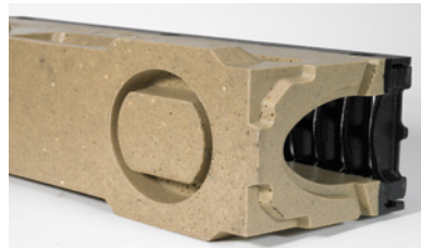
ACO DRAIN® PowerDrain V 75/100 P 0,5 m varauksella poistoyhteelle (knock out)
